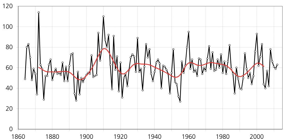
Abbildung 3.5: Jährliche Anzahl Beobachtungstermine mit Föhn an der Station Altdorf in der Periode 1864-2012. Beobachtungstermine sind 07:00 h, 13:00 h sowie 21:00 h (ab 1971 19:00 h). Die ausgezogene Linie zeigt das über 20 Jahre gleitende Mittel (Gauss-Tiefpassfilter).
