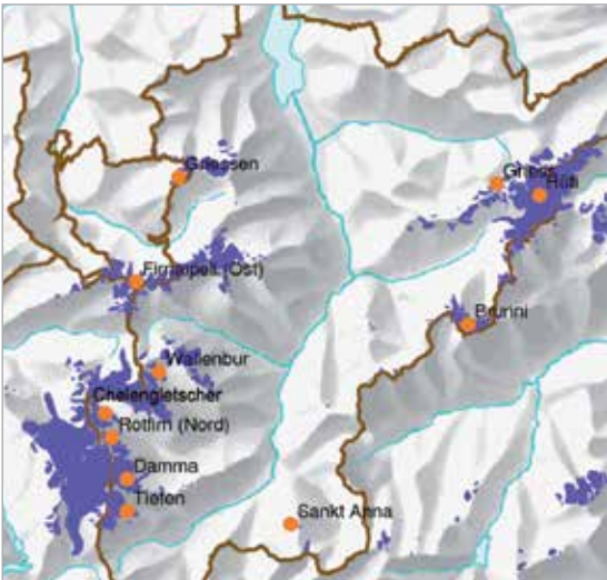
Abbildung 4.10: Vergletschertes Gebiet der Urschweiz mit Gletschern aus dem Schweizer Gletschermessnetz (weitere Kennzahlen sind der Tabelle 4.2 zu entnehmen).
