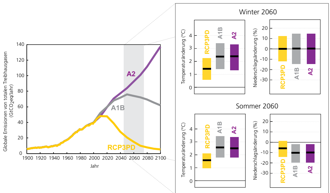
Abbildung 5.1: Totale globale anthropogene Treibhausgasemissionen der drei in diesem Bericht berücksichtigten IPCC Emissionsszenarien RCP3PD (gelb), A1B (grau) und A2 (lila) für die Jahre 1900-2100 und projizierte Urschweizer Temperatur- (°C) und Niederschlagsänderungen (%) für „2060“ (das Mittel der Periode 2045-2074) gegenüber 1980-2009 im Winter (oben) und Sommer (unten).
