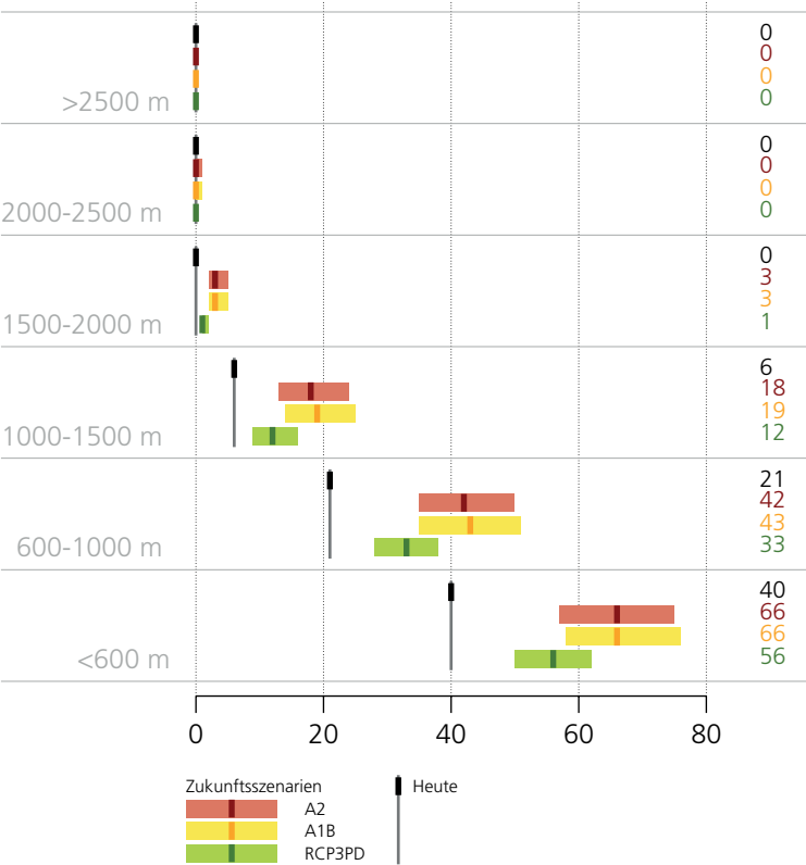
Abbildung 5.4: Die Anzahl Sommertrage pro Kalenderjahr heute (Mittel 1980-2009) und 2060 (Mittel 2045-2074) für die drei Szenarien A2, A1B und RCP3PD und 6 Höhenstufen (<600, 600-1000, 1000-1500, 1500-2000, 2000-2500 und >2500 m ü.M.). Die Abschätzung basiert auf der projizierten Temperaturänderung im Alpenraum (Zubler et al. 2013). Die Zahlen und Balken geben die mittlere Schätzung und den Unsicherheitsbereich der Modellschätzungen wieder.
