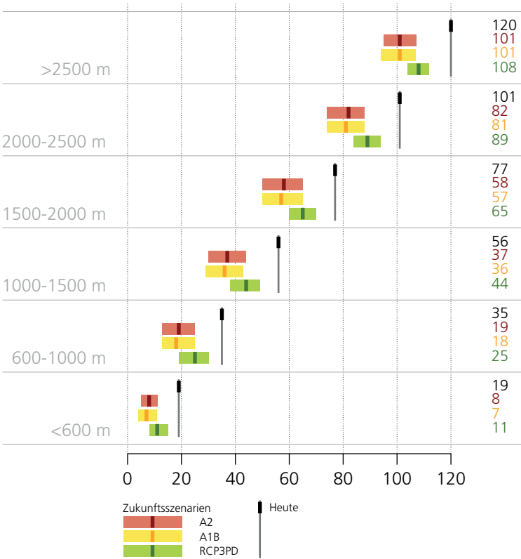
Abbildung 5.6: Die Anzahl Tage mit Neuschnee pro Kalenderjahr heute (Mittel 1980-2009) und 2060 (Mittel 2045-2074) für die drei Szenarien A2, A1B und RCP3PD und 6 Höhenstufen (<600, 600-1000, 1000-1500, 1500-2000, 2000-2500 und >2500 m ü.M.). Die Abschätzung basiert auf der projizierten Temperaturänderung im Alpenraum (Zubler et al. 2013). Die Zahlen und Balken geben die mittlere Schätzung und den Unsicherheitsbereich der Modellschätzungen wieder.
